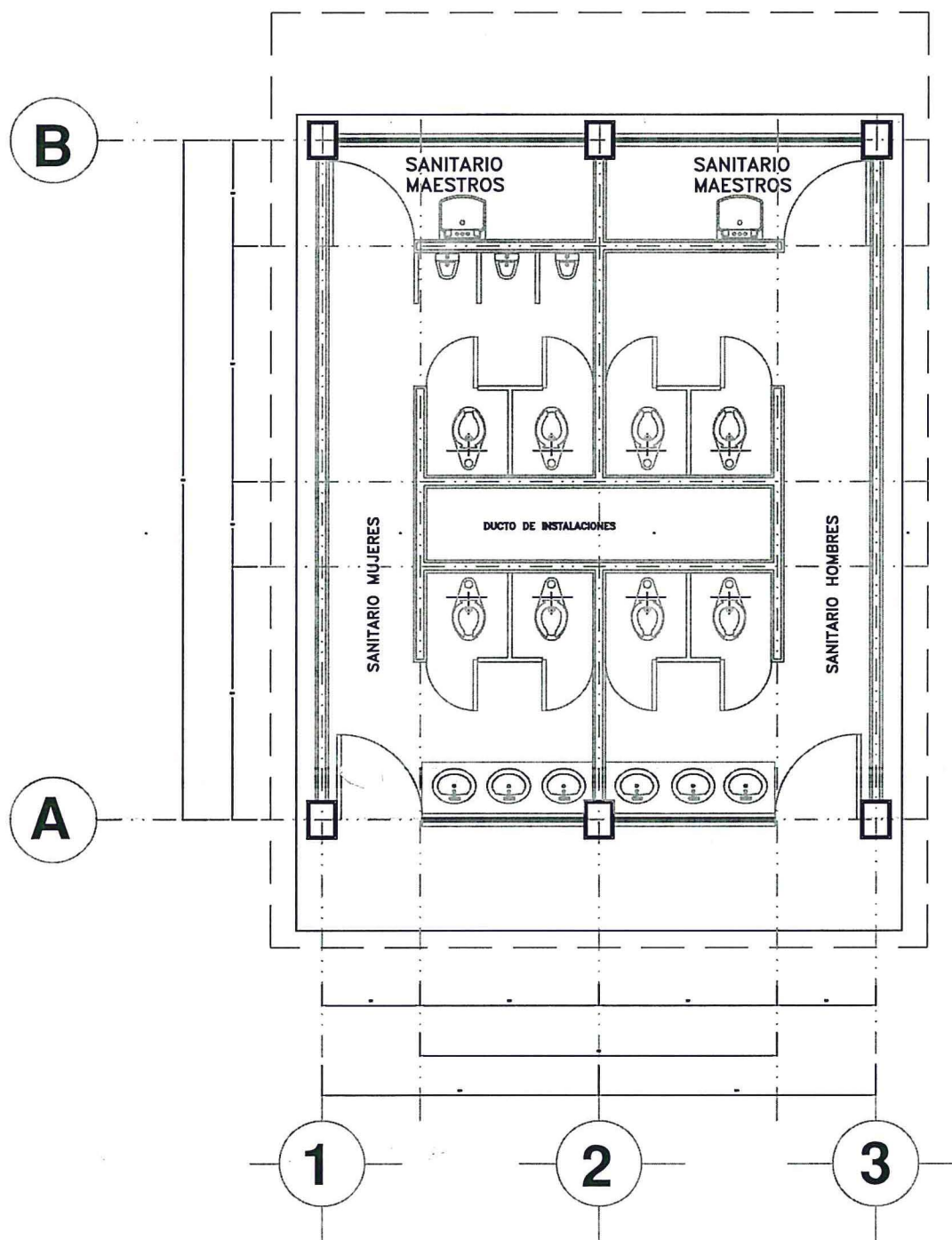
PLANTA TIPO SERVICIOS SANITARIOS
